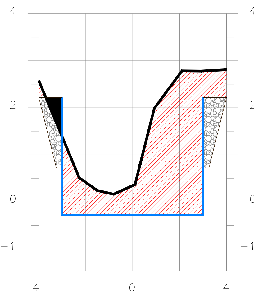
SECCION 2+415
