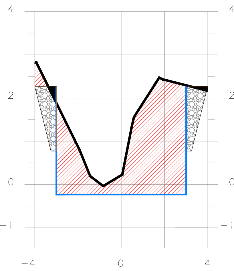
SECCION 2+295
