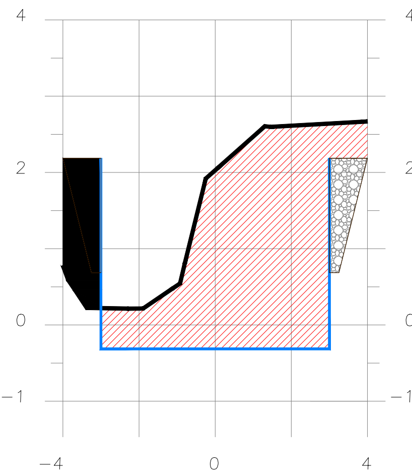
SECCION 2+490
