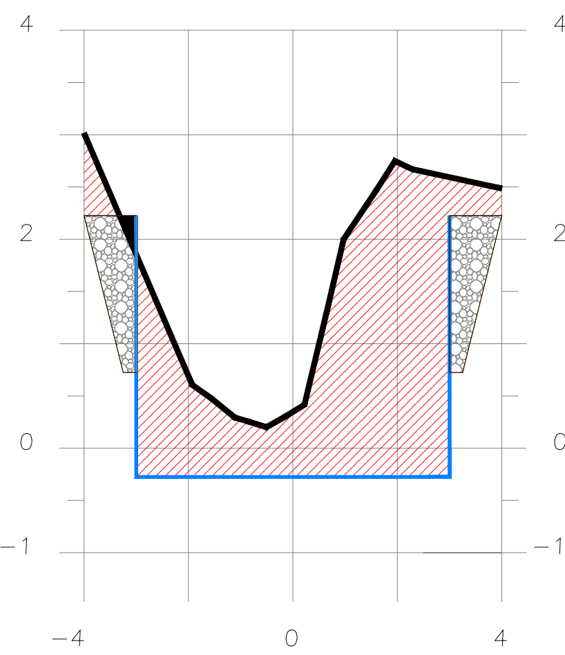
SECCION 2+400
