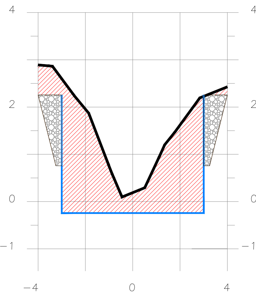
SECCION 2+325
