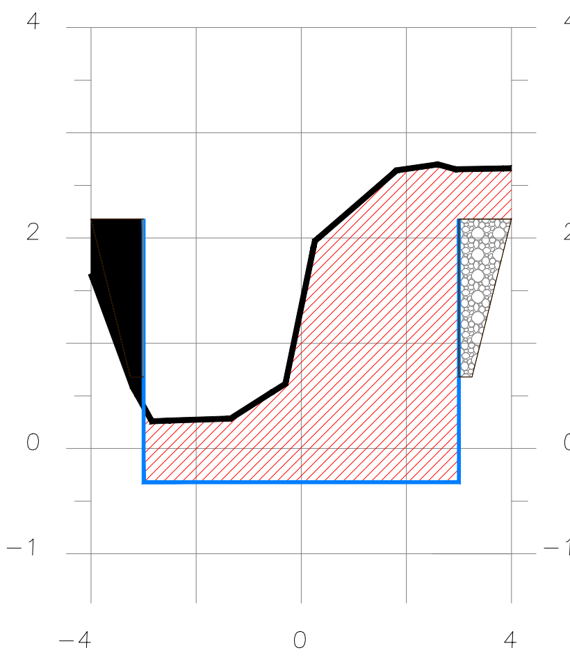
SECCION 2+505
