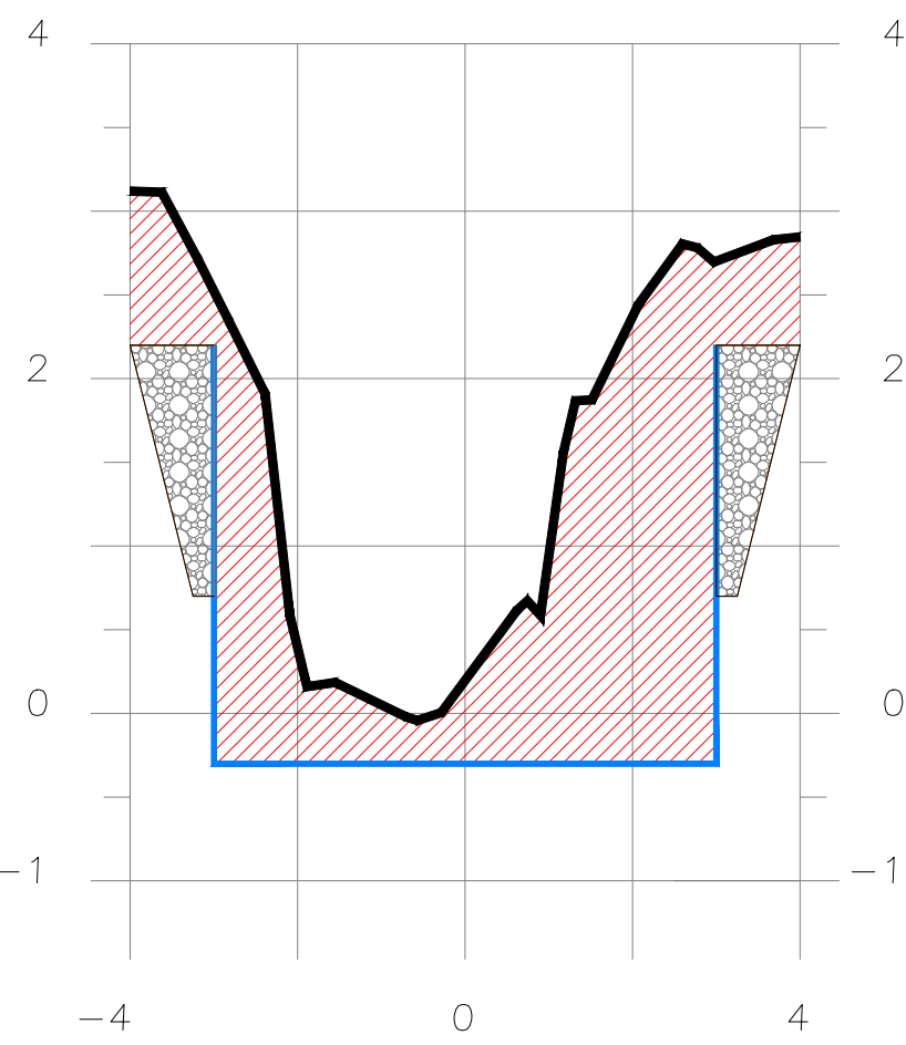
SECCION 2+460
