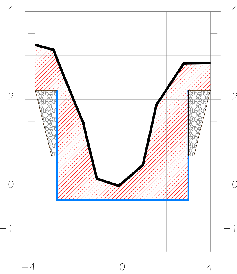
SECCION 2+445
