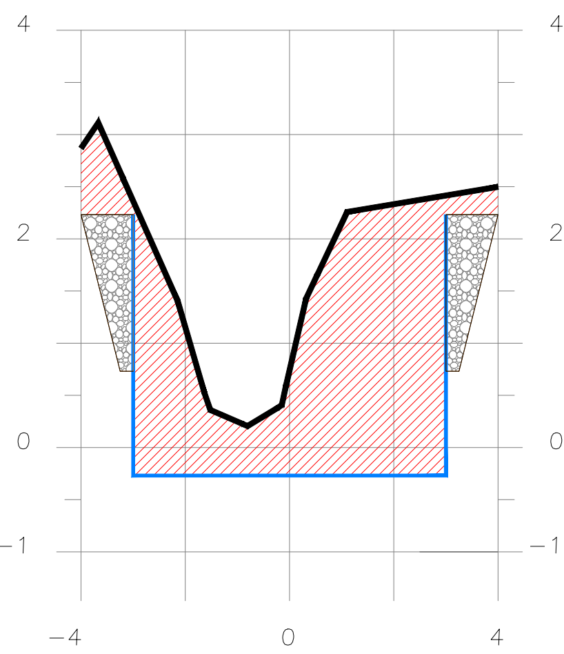
SECCION 2+385
