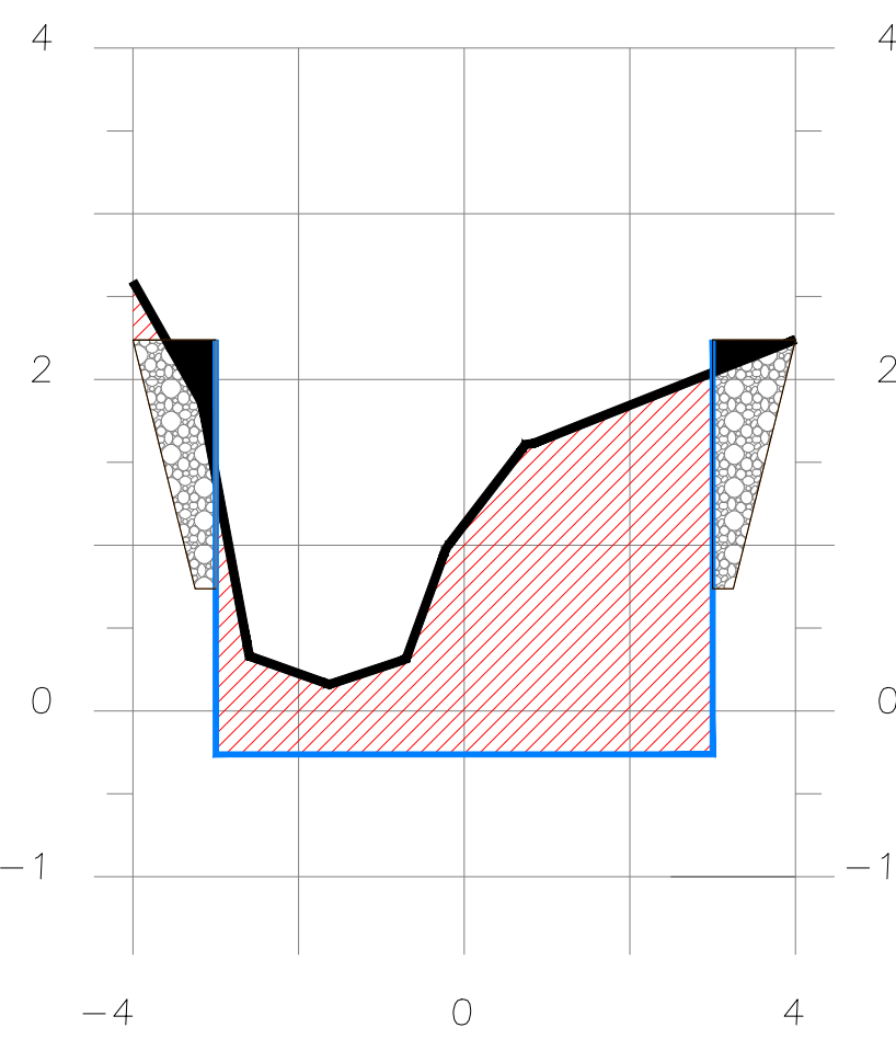
SECCION 2+370
