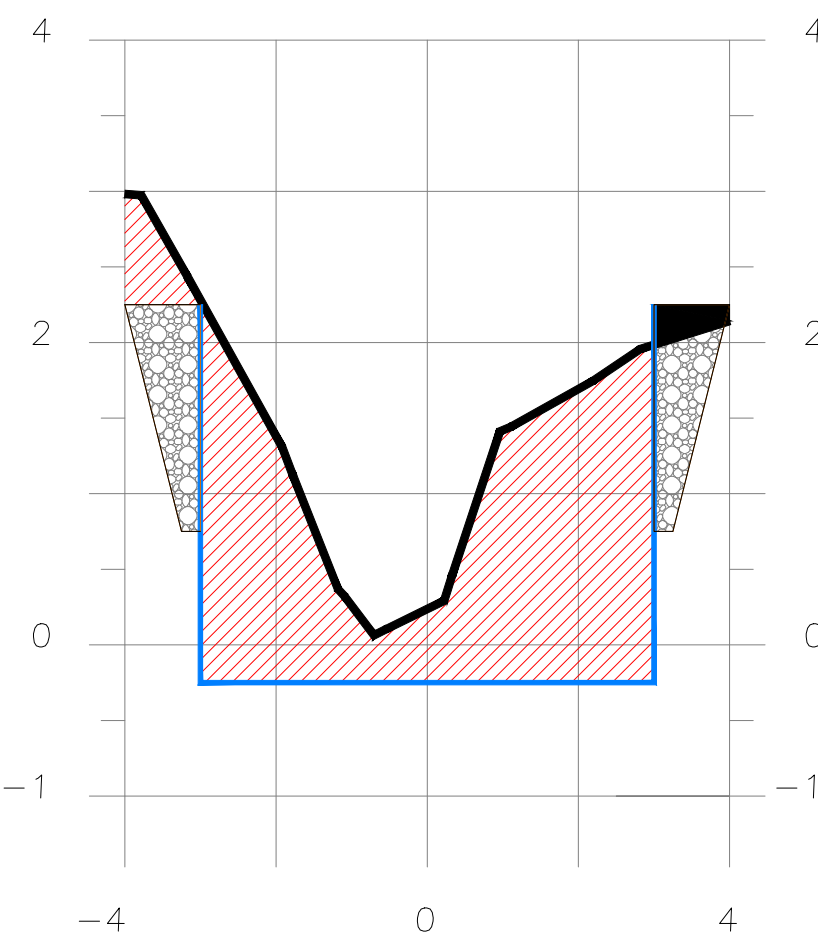
SECCION 2+340
