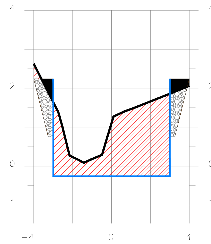
SECCION 2+355
