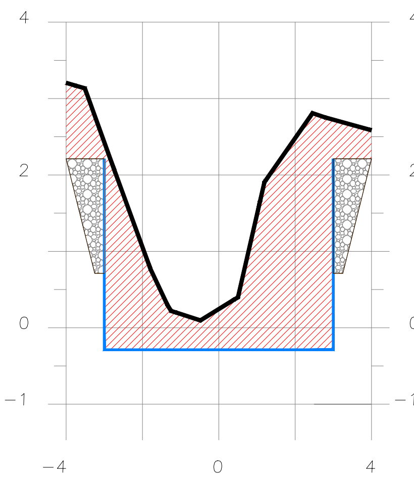
SECCION 2+430
