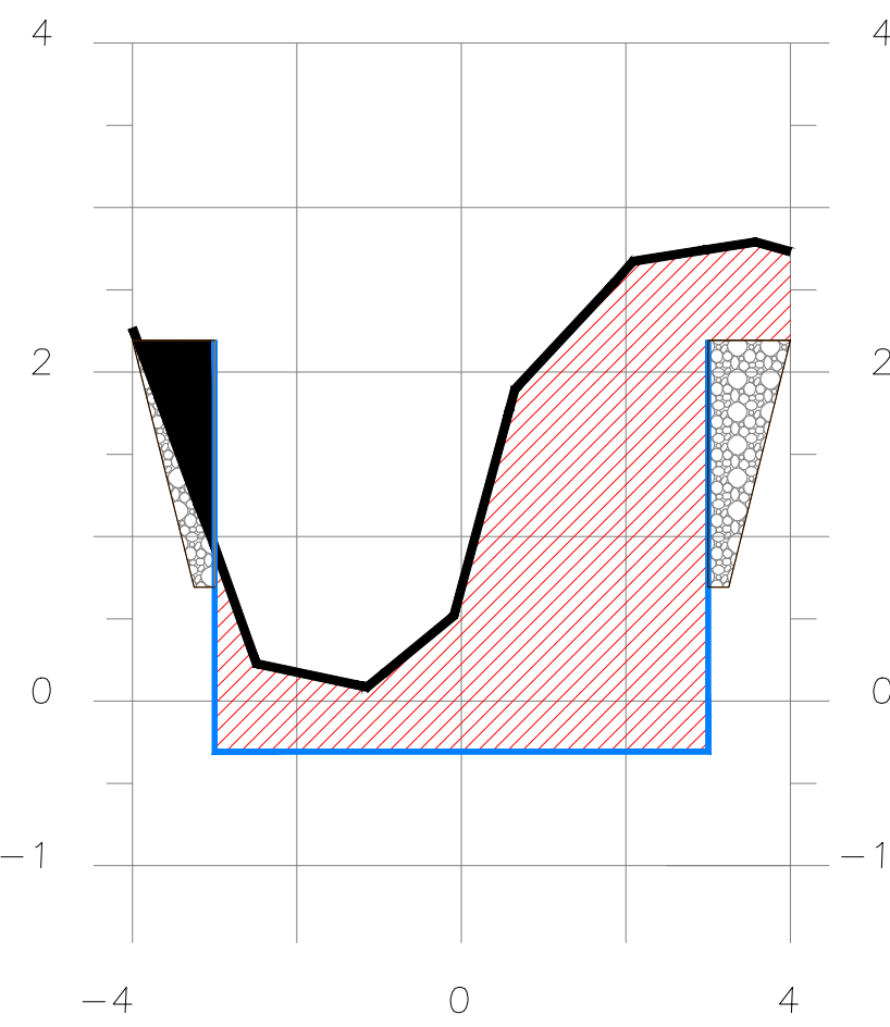
SECCION 2+475
