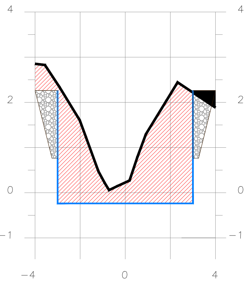
SECCION 2+310
